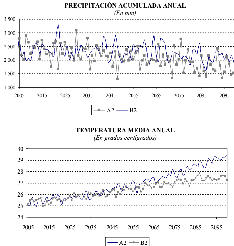
Gráfico III-1 ISTMO CENTROAMERICANO: ESCENARIOS A2 PROMEDIO Y B2 PROMEDIO
