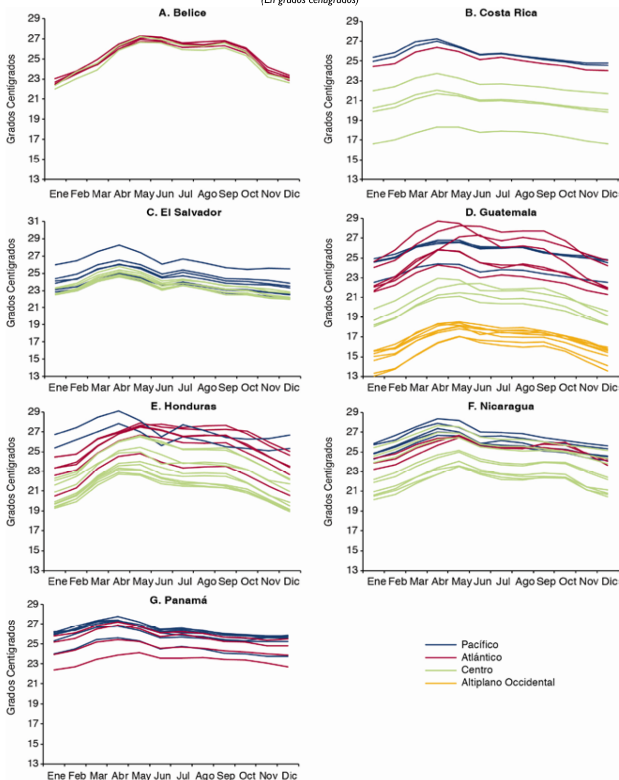
GRÁFICO 7 CENTROAMÉRICA: TEMPERATURA MEDIA MENSUAL POR PAÍS, DEPARTAMENTO Y REGIÓN GEOCLIMÁTICA, PROMEDIO 1950 – 2000 (En grados centígrados)
