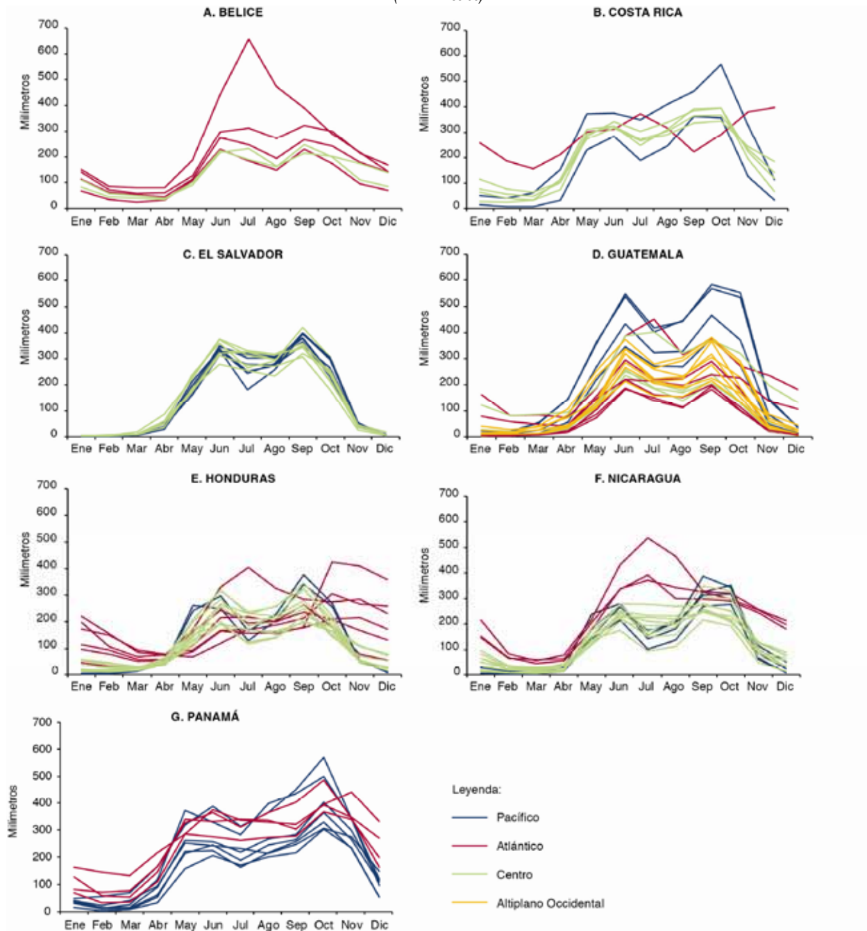
GRÁFICO II CENTROAMÉRICA: PRECIPITACIÓN MENSUAL POR PAÍS DEPARTAMENTO Y REGIÓN GEOCLIMÁTICA, PROMEDIO 1950-2000 (En milímetros)
