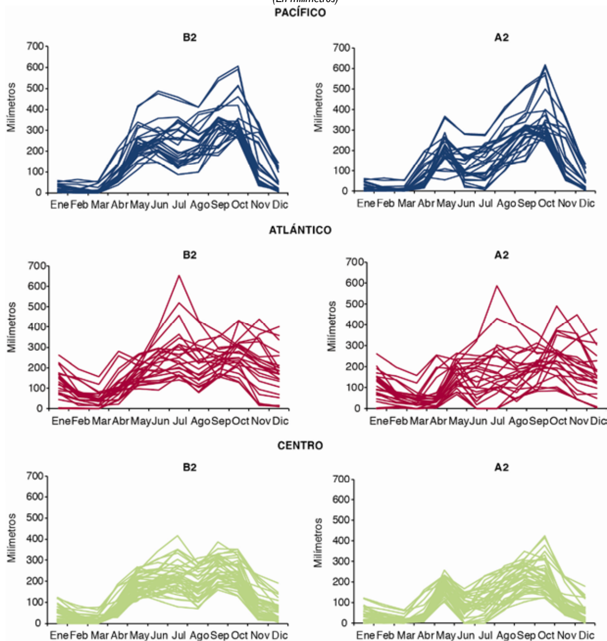
GRÁFICO 18 CENTROAMÉRICA: PRECIPITACIÓN MENSUAL POR DEPARTAMENTO Y REGIÓN GEOCLIMÁTICA (DESAGREGADO), ESCENARIOS B2 Y A2, 2100
