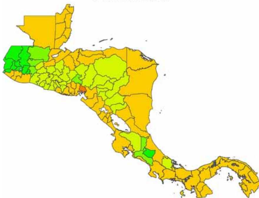
MAPA 4 (AMPLIACIÓN) CENTROAMÉRICA: TEMPERATURA MENSUAL MEDIA ANUAL POR DEPARTAMENTO, ESCENARIO A2, PROMEDIO 1950-2000 Y 2100 (En grados Centígrados) A. PROMEDIO 1950-2000
