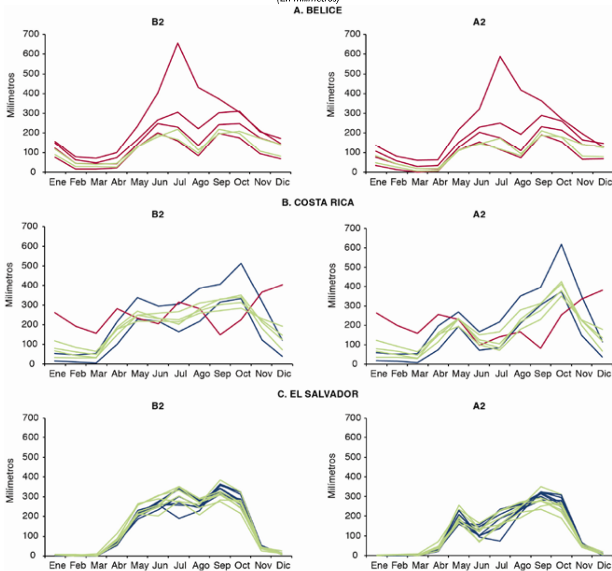
GRÁFICO 19 CENTROAMÉRICA: PRECIPITACIÓN MENSUAL POR PAÍS, DEPARTAMENTO Y REGIÓN GEOCLIMÁTICA, ESCENARIOS B2 Y A2, 2100 (En milímetros)
