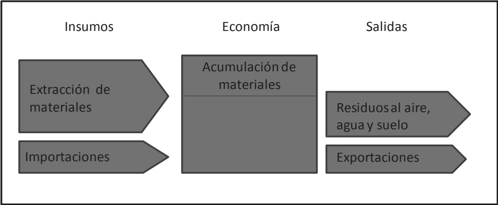
Figura 1 Esquematzación del flujo de materiales en un sistema socio-económico.
