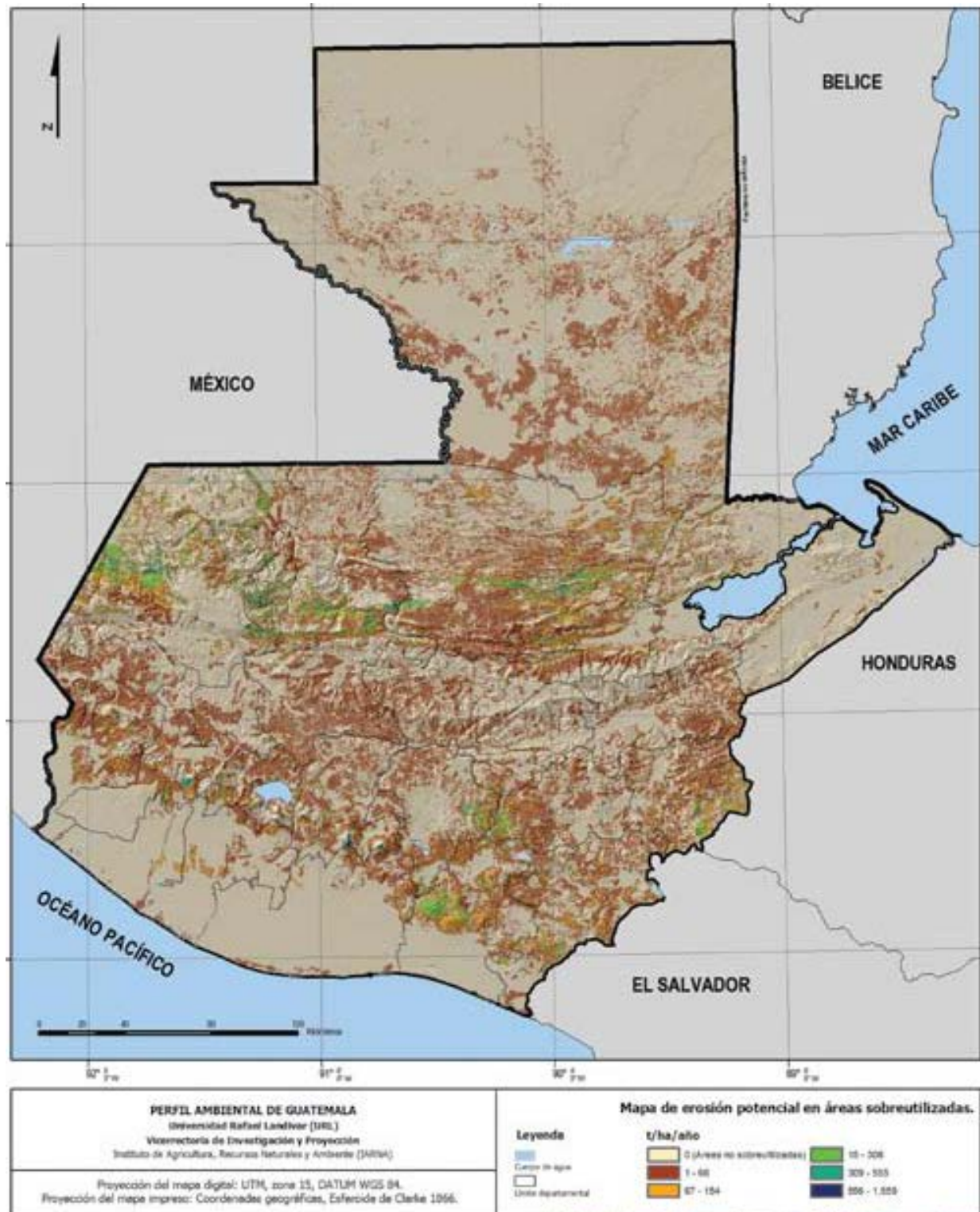
Figura 27. Erosión potencial en Guatemala en t/ha/año para áreas con sobreuso
