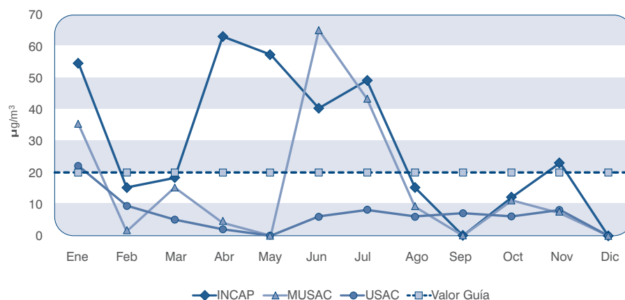
Gráfica 2.5 Guatemala: Dióxido de azufre ( \text{SO}_2 ) en la ciudad de Guatemala 2009 (Promedio mensual en \mu\text{g}/\text{m}^3 )
