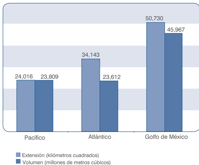
Gráfica 1.2 Guatemala: Superficie de las vertientes y volumen de agua por vertiente 2006 (km² y millones de metros cúbicos)
