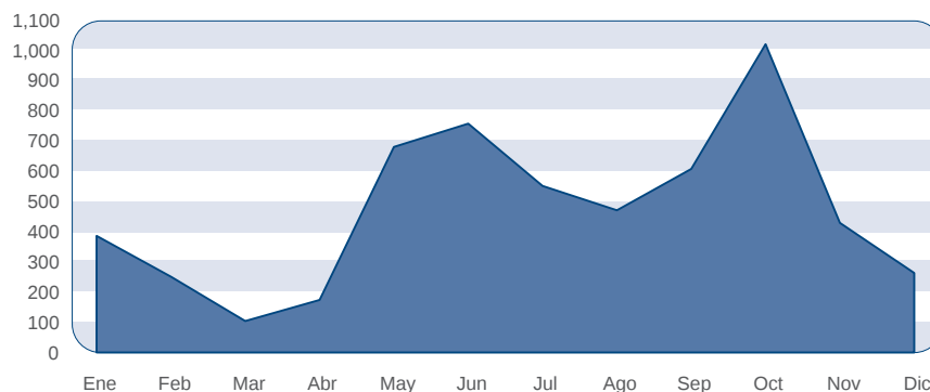
Gráfica 2.7 Guatemala: Precipitación pluvial anual 2009 (Milímetros)
